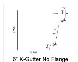
6" K-Gutter No Flange
