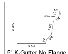
5" K-Gutter No Flange
