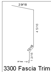
3300 Fascia Trim
