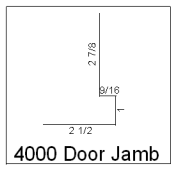
4000 Door Jamb
